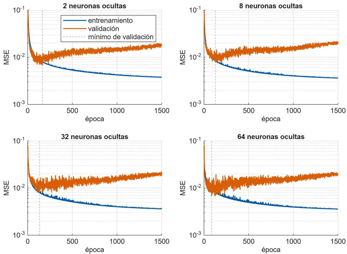
Figura 5: Error de entrenamiento y de validación sobre Breast Cancer para cuatro anchos de capa oculta. La línea discontinua marca la época de mínimo error de validación
