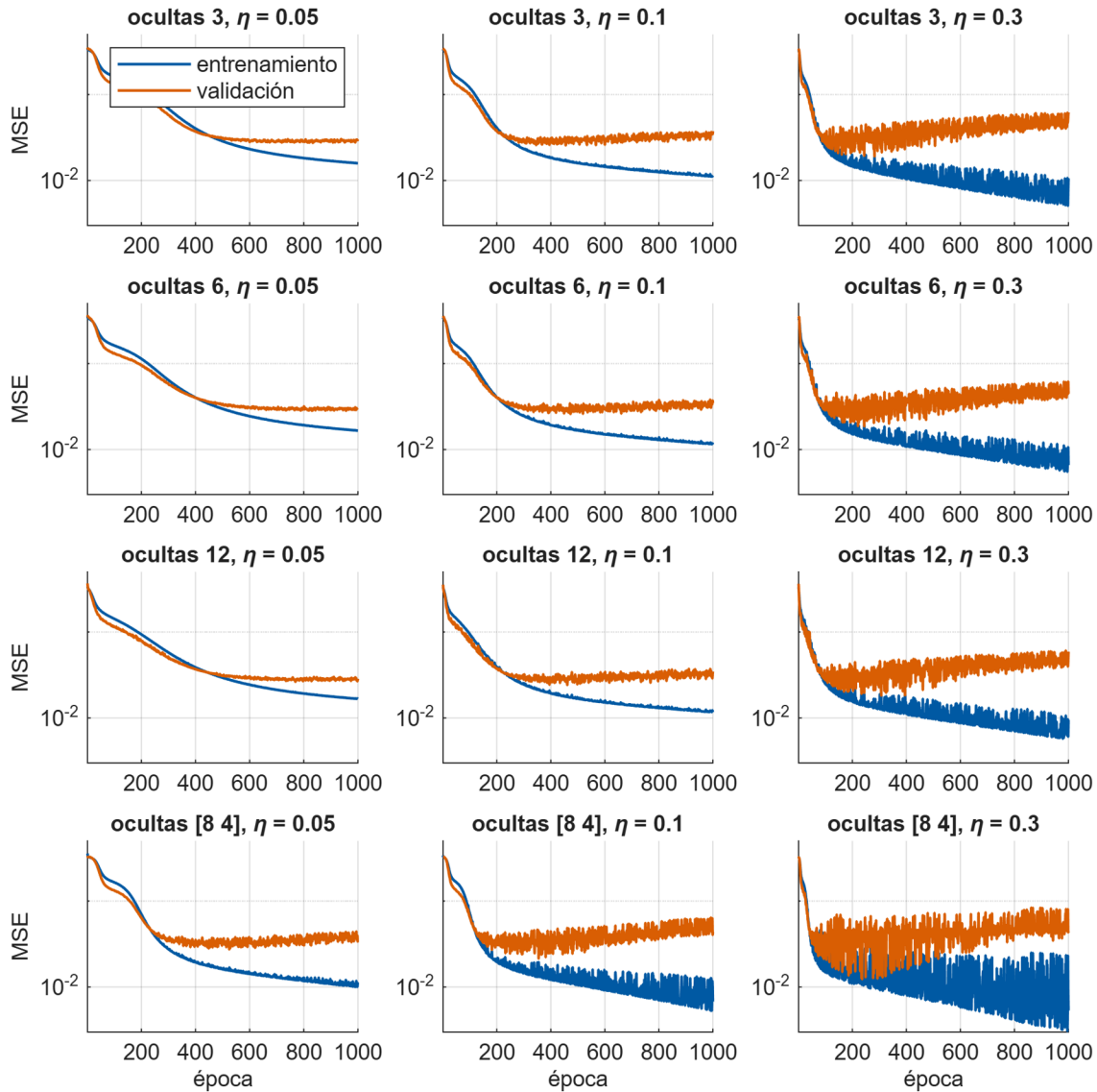
Figura 3: Curvas de error de entrenamiento y de validación sobre Iris para las cuatro arquitecturas y las tres tasas de aprendizaje, en escala logarítmica
