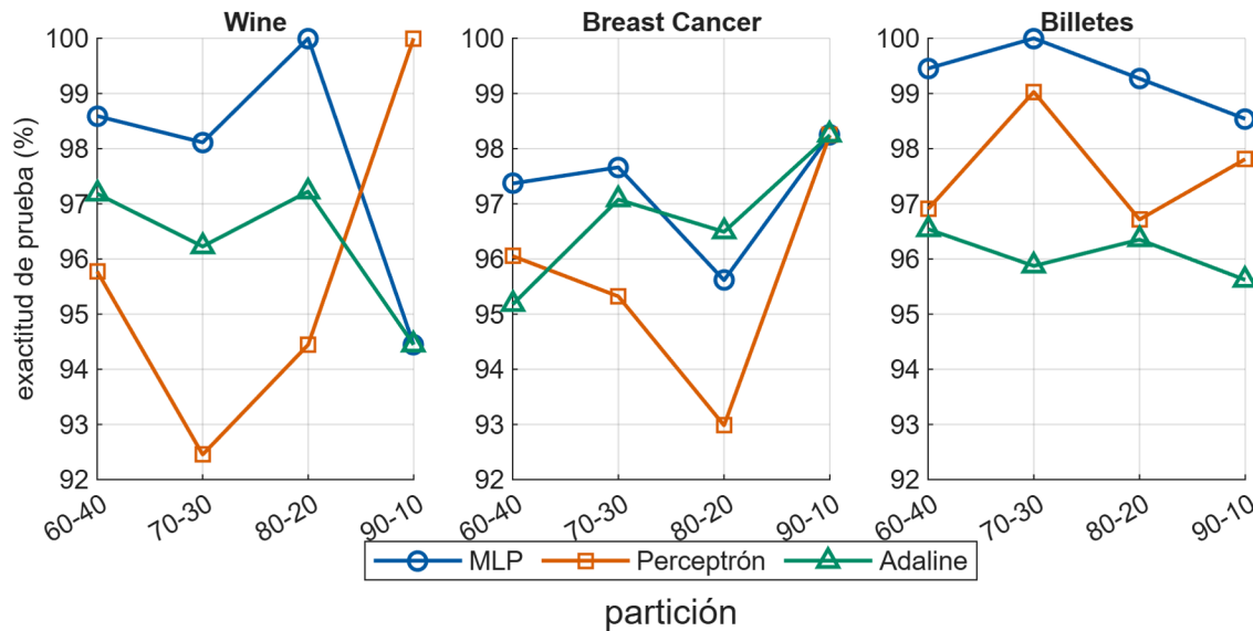
Figura 4: Exactitud de prueba de los tres modelos según la proporción de partición en los tres conjuntos reales, con el mismo rango vertical en los tres paneles
