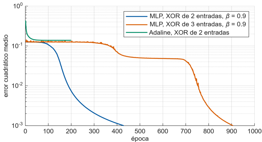
Figura 1: Curva de error de entrenamiento sobre la XOR. El MLP con cuatro neuronas ocultas y momento 0.9 llega al error objetivo, el Adaline se estanca cerca de 0.139, apenas por encima del piso de 0.125 de la mejor función lineal
